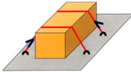
Amarração Vertical (por Atrito)
